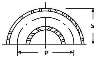
180° L.R. Return
