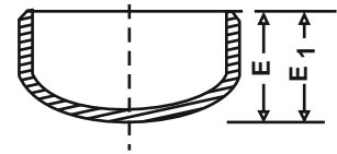
CAP
