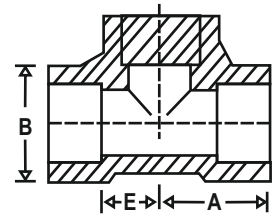
TEE
